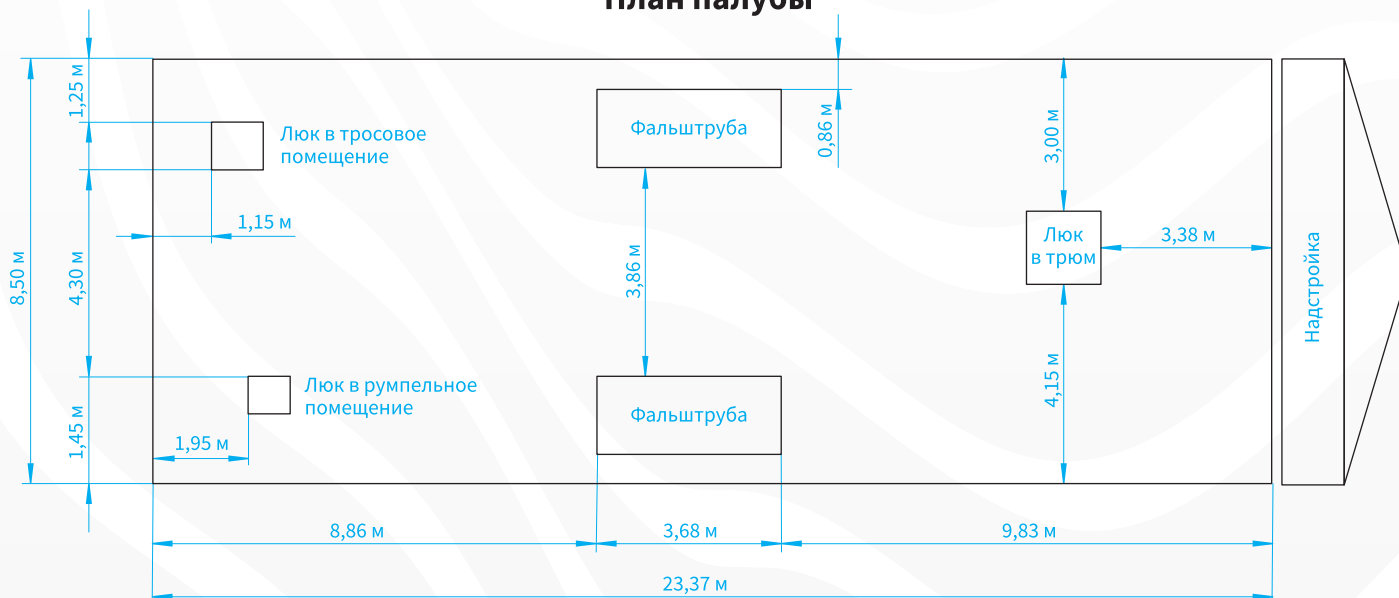
План палубы
