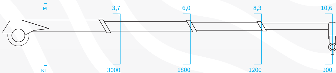
Грузоподъёмность крана СФ-125 на различном вылете стрелы с лебёдкой
